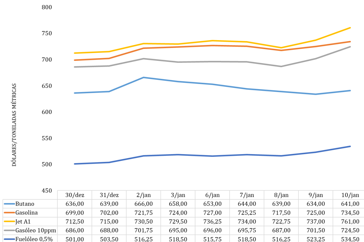
Gráfico 2 – Preços dos derivados de petróleo
